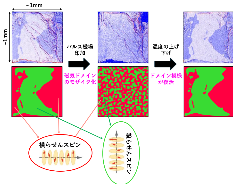
図3：無磁場で観測された、らせん状スピン秩序の磁気ドメイン構造とその柔軟な応答性
