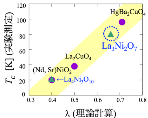
図2 理論計算と実験測定データの相関関係。 三角形が本研究で調べた物質( \text{La}_3\text{Ni}_2\text{O}_7 , \text{La}_4\text{Ni}_3\text{O}_{10} )を指す。 円形は一層型の超伝導体を指す。
