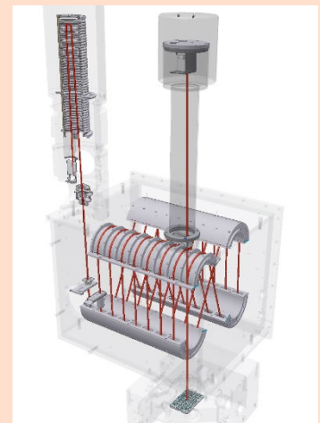
阪大で開発されたMULTUMイオン光学系を応用して開発されたJMS-S3000のイオン軌道図
