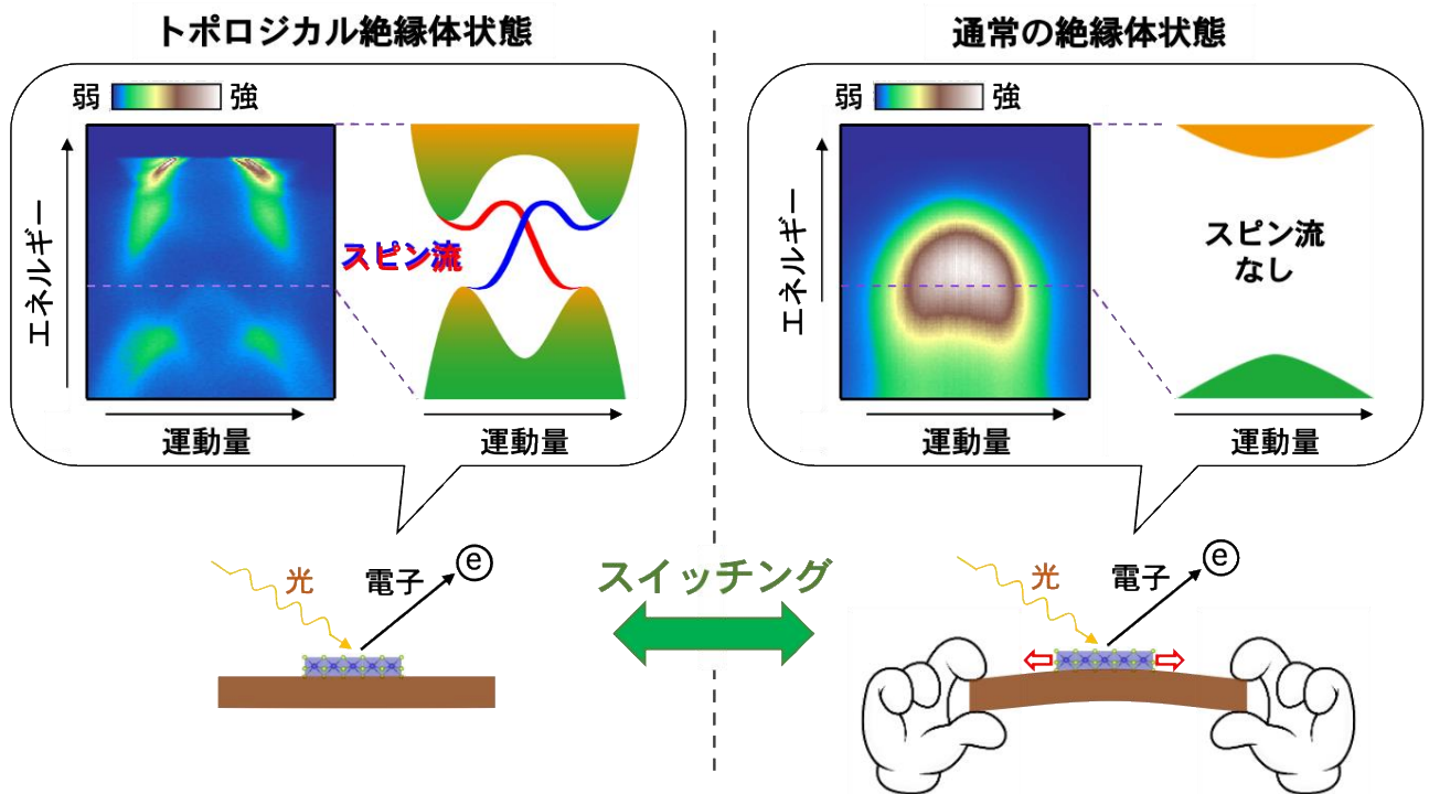
図2：物質内を一見乱雑に動き回る電子の振る舞いも、電子1つ1つを運動量とエネルギーの関係（電子構造）としてプロットするとすっきりと整理される。これは量子力学に従う電子ならではの性質である。この電子構造の様子は物質それぞれの個性を示し、それが解明できるとあらゆる電氣的・磁氣的な性質が理解できる。本研究で利用した角度分解光電子分光は、物質の電子構造を直接的に決定できる実験手法である。また電子が持つスピンの向きを同時に測定することで、スピン流の微視的な振る舞いを可視化することが可能となる。本研究では、これらの実験技術を駆使して、擬一次元 TaSe 3 がトポロジカル絶縁体状態にありスピン流を生成することを初めて解明した（左図）。また、TaSe 3 が固体の中でも柔らかい物質である利点を生かし、基板を少し曲げて試料に歪みを生じさせることで、通常絶縁体へと変化させられることを、電子構造の観察から実証した（右図）。左図に、試料に歪みを生じる前の電子構造を、実験データおよび模式図で示す。また、右図には、基板を曲げて試料に張力歪みを生じさせると電子構造が激変した結果を、実験データと模式図で示す。この変化と共にスピン流が消失したことは、対応する電子構造の強度が消失していることから理解できる。
