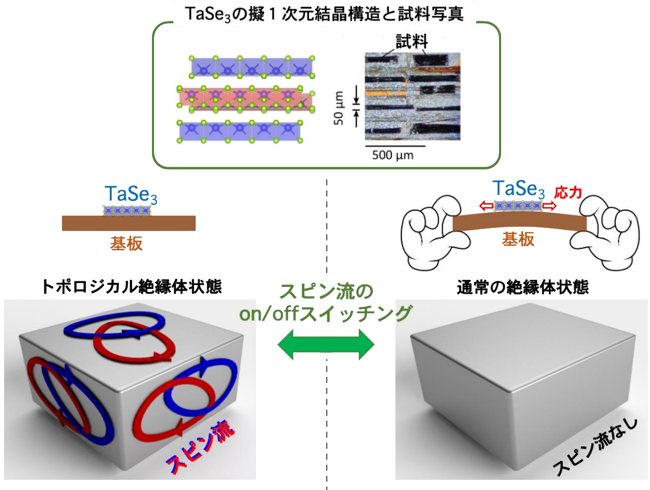
図 1 : (上図) TaSe 3 は、鎖状の構造が積み重なって形成されるため、擬一次元的な結晶構造と電気伝導を示す。(左下図) 外から歪みを加えない状態の TaSe 3 はトポロジカル絶縁体状態となり、結晶の表面にスピンの流れが生成されることが分かった。(右下図) 基板に試料を乗せ、それをたわませると、赤い矢印方向に応力が印加され試料に歪みが生じる。その結果、TaSe 3 は通常の絶縁体となりスピンの流れが消失する。基板をたわませる・たわませないの簡単な操作で、スピンの on/off スwitching が可能となる。
