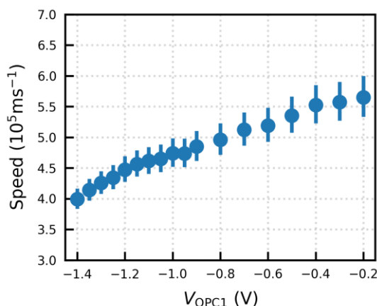
図 2: QPC の閉じ込め幅に依存したプラズモン波束の速度。横軸に沿った QPC における回路幅の部分的な変調によって、プラズモン波束の速度が制御される様子を示している。
