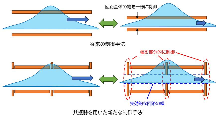
図 1: 従来の固有状態制御手法と本研究で開発した新手法の比較。従来の手法では、プラズモン波束(水色)が通過する回路全体の幅を一律に制御していました。回路の幅が広いとプラズモン波束の速度は大きく、幅が狭いと小さくなります。共振器を用いた新たな手法では、部分的に幅を制御することで、回路全体の実効的な幅を狭くする効果を得ることができます。
