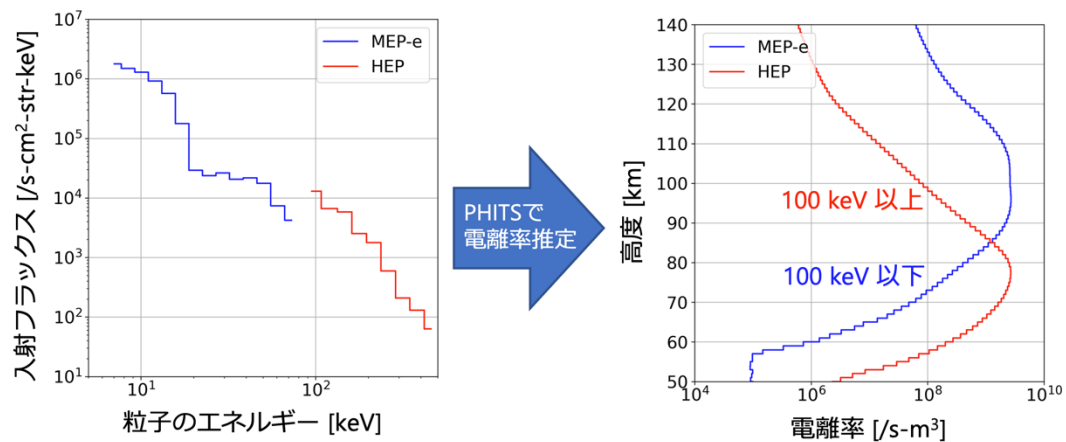
図3：「あらせ」衛星による降下電子のフラックスの観測結果(左)を入力とした、電離率の推定結果(右)。
