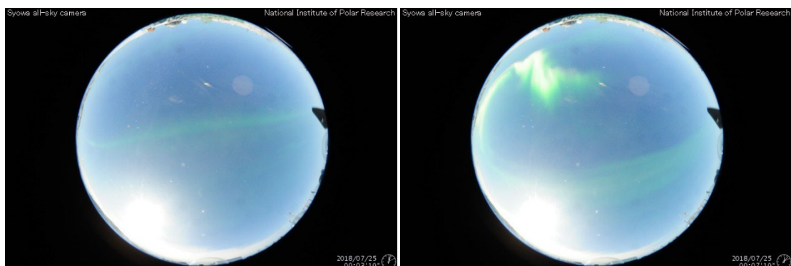
図 2：世界時 注5 2018 年 7 月 25 日 0 時 5 分前後のオーロラの様子(注：視野の左下は月明かり)。左は、低高度で大気電離が観測されていたオーロラ爆発 2 分前。右はオーロラ爆発時で、このとき低高度の大気電離は見られなかった。（提供：国立極地研究所・宮岡宏）
