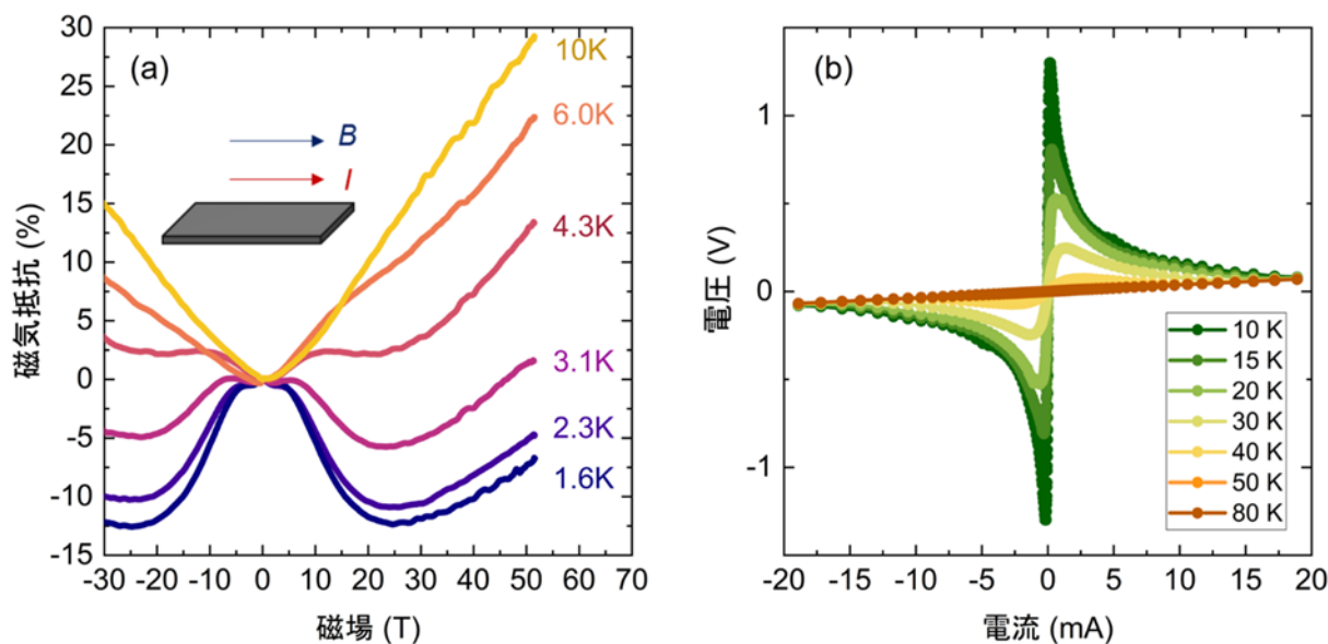
図3 \alpha -(BETS) 2 I 3 の特異な磁場・電場応答性
