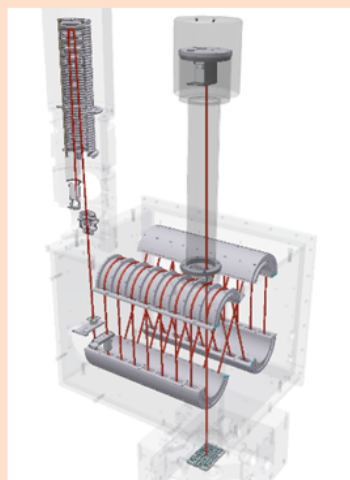
阪大で開発されたMULTUMイオン光学系を応用して市販化されたJMS-S3000のイオン光学系
