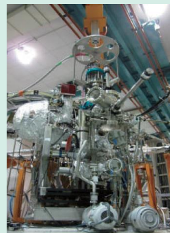
固体の電子状態をつぶさに観測できる三次元運動量・軌道対称性分解光電子分光装置。
