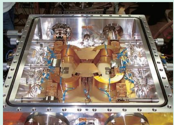
当グループで開発したマルチターン飛行時間型質量分析計「MULTUM Linear plus」。
