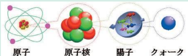
原子、原子核、核子の階層構造
