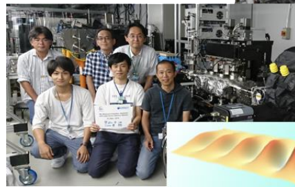
プラズマ中のレーザー航跡場
