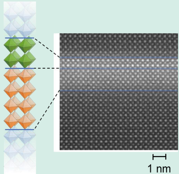
3種類の強相関酸化物を積層して合成した界面構造
