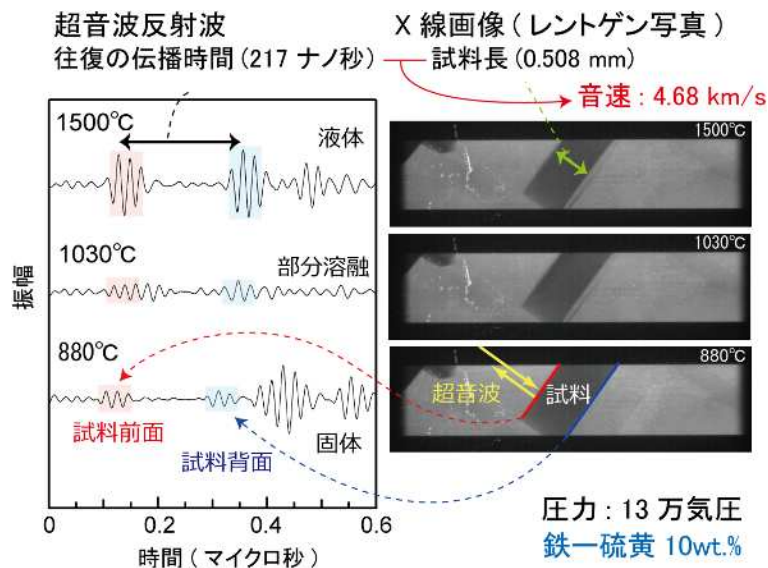
図1 : 13 万気圧における、鉄-10wt%硫黄合金(Fe 80 S 20 )の超音波信号と X 線画像
