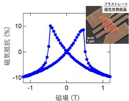
図 1: 本研究で得られた巨大磁気抵抗と素子の電子顕微鏡像。
