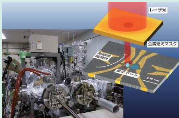
半導体高品質成膜装置(左)と量子ドットを使った光子-電子スピン結合(右)
