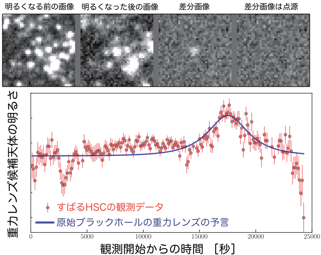
図3 今回のすばる HSC のアンドロメダ銀河のデータから見つけた、たった一つの原始ブラックホールによる重力マイクロレンズ効果の候補天体。横軸は 2014 年 11 月 23 日の観測開始時間からの時間（秒単位）、縦軸は候補天体の明るさ。観測開始から約 14,000 秒（約 4 時間）後に星が徐々に明るくなり、約 17,000 秒後（約 4 時間 40 分後）に最大の明るさになり、その後徐々に暗くなった（元の星の明るさに戻った）ことを示す。実線は、この観測結果を再現する重力マイクロレンズ効果の予言。上の画像は、候補天体の画像。左から右にかけて、候補天体の明るくなる前の画像、明るくなった後の画像、その 2 つの画像の差分画像（明るさが変わらないまわりの星は消えている）。明るさの変化した星の明るさ変化のみが示されており、差分画像から明るさ変化した天体が点源（星）であること（不正確な解析による系統誤差、間違いではないこと）を示している（Credit : Niikura et. al）。
