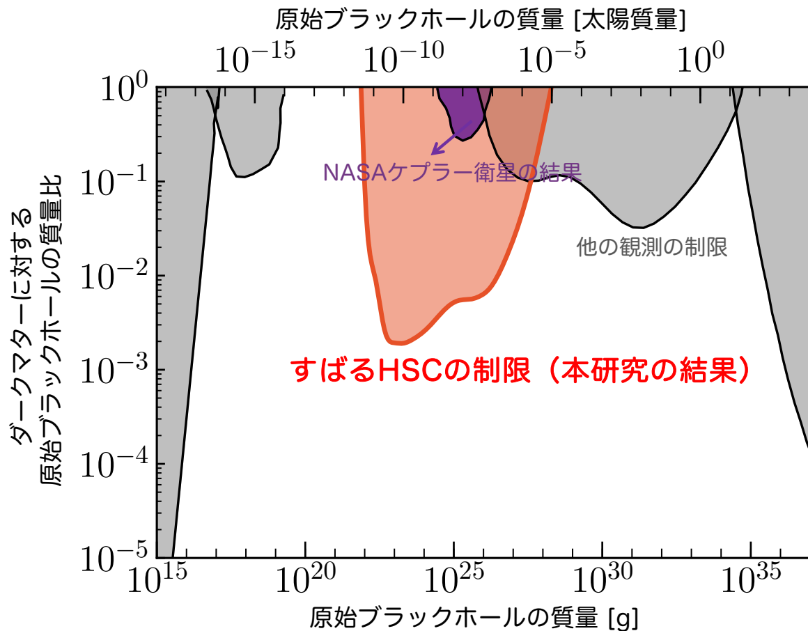
図4 オレンジ色の塗られた領域は、本研究の重力マイクロレンズ効果の探索から得られた、原始ブラックホールの存在量の制限（塗られた領域は許されない領域）。横軸は原始ブラックホールの質量（下側の数値の単位はグラム（g）、上側の数値は太陽質量の単位）、縦軸は天の川銀河とアンドロメダ銀河のあいだに存在するダークマターの総量に対する原始ブラックホールの質量比。縦軸が1（10の0乗）の場合は、すべてのダークマターが原始ブラックホールである場合に対応する。他のグレーの領域は他の観測による制限。本研究のたった1晩のHSCのデータを使った解析から、NASAのケプラー衛星の2年間のデータよりも厳しい制限が得られたのが分かる（Credit：Niikura et. al）。
