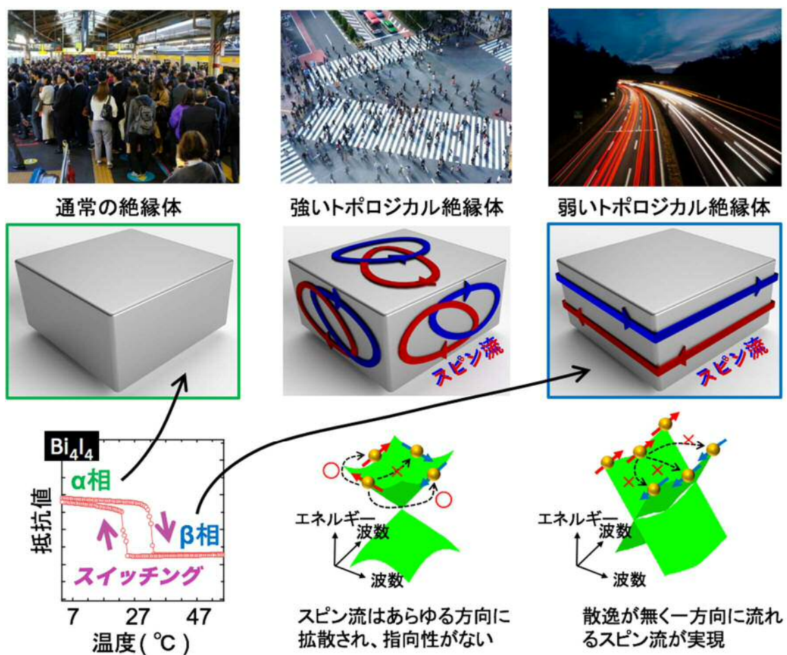
図 1：通常の絶縁体と「強い」・「弱い」トポジカル絶縁体の概略図。通常の絶縁体で
