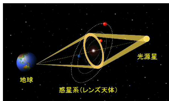
図3: 重力マイクロレンズによる系外惑星検出の概念図
