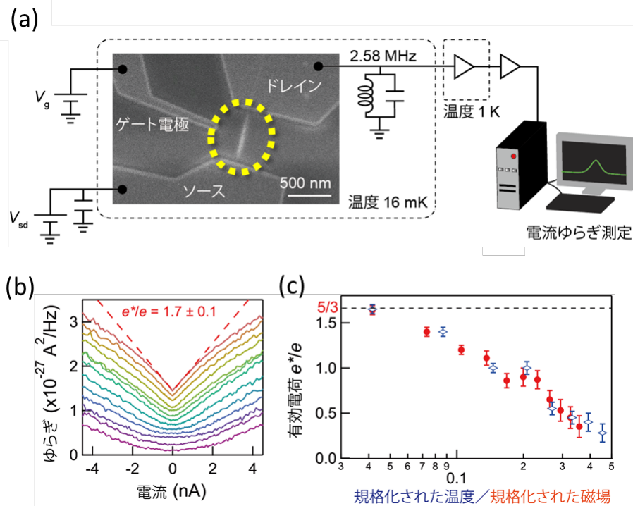
図 2: (a) 実験に用いた試料の電子顕微鏡写真および測定回路の概略図。黄色い点線で囲まれた領域に見える白い筋が、カーボンナノチューブからなる人工原子です。この人工原子にただひとつの電子を閉じ込め、それによって生じる近藤効果を、電流と電流ゆらぎ測定によって解析しました。(b) 得られた実験結果。縦軸は電流ゆらぎの大きさ、横軸は、人工原子に形成された近藤状態によって跳ね返される電流の大きさを示しています。様々な磁場でゆらぎ測定を行った結果、有効電荷 e^*/e が 1.7 と求まりました。(c) 有効電荷が、近藤温度や磁場によってスケールされる様子を示します。このような非平衡状態におけるスケールリングは、本研究によって初めて明らかになりました。
