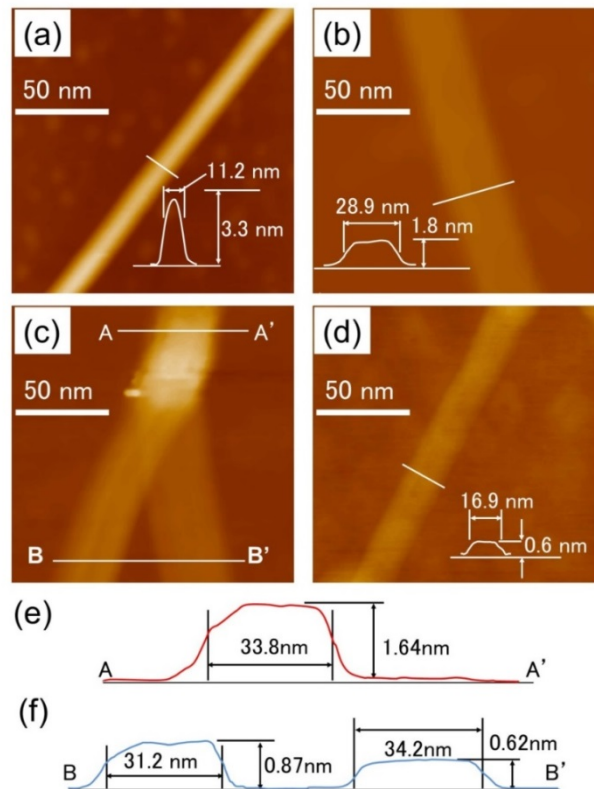
図2. AFM 像 (a) 出発物質のDWNT (b) アンジップで得られたdGNR (c) 2枚のGNRが剥がれて別々のsGNRになろうとしている領域。(d) 得られたsGNR. 各々のスケールバーは50nm。(e) (c)中のdGNRのラインプロファイル。(e) (c)中のdGNRのラインプロファイル。(a), (b), (d)中のラインプロファイルは図中の線に沿って得られた。(a)-(d)は別の試料で得られた結果である。
